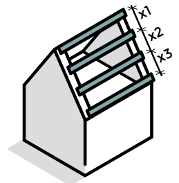
MEERVELDS OVERSPANNING
