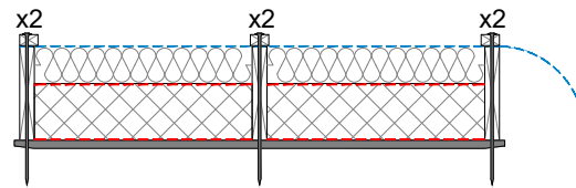
Stap 3: Afgewerkt mini-element waarmee de gewenste dakbreedte bereikt wordt
