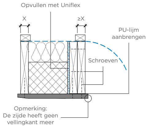
Stap 1: Element aanpassen naar gewenste breedte
